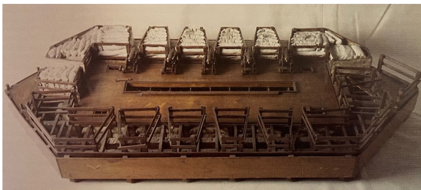
Maqueta de las baterías flotantes diseñadas por Michel D'Arçon para el «Gran Sitio de Gibraltar».
